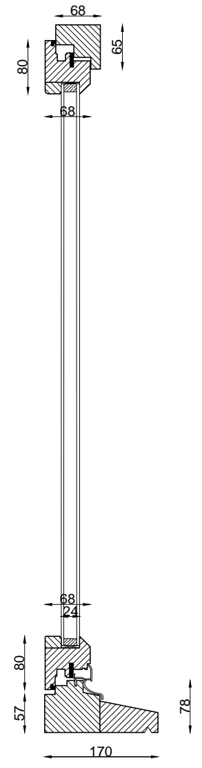
Section A-A
